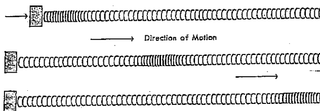
Longitudinal wave
